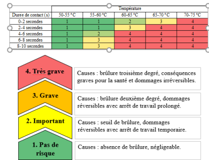
Figure 9 : Passage du tableau des valeurs thermiques à une échelle à trois niveaux
