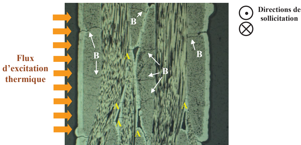
Figure 5 – Cliché micrographique du composite étudié post-essai Mise en évidence de la fissuration transverse (A) et matricielle (B)
