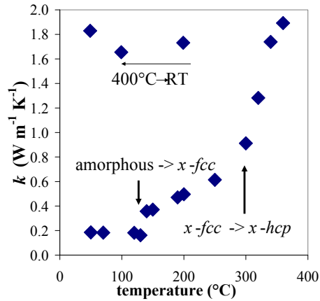
Figure 1 : Conductivité thermique du \text{Ge}_2\text{Sb}_2\text{Te}_5 mesurée par radiométrie photothermique modulée sur la plage de température 50 - 400 ^{\circ}\text{C} .
