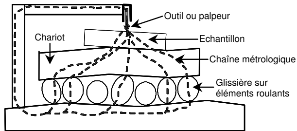
Fig. 4. – Structure classique.
